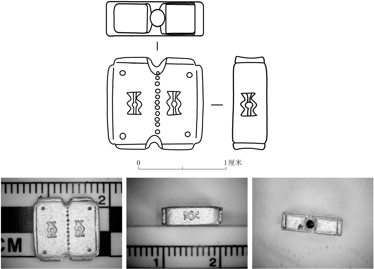
图一三 方形串饰M1:26
